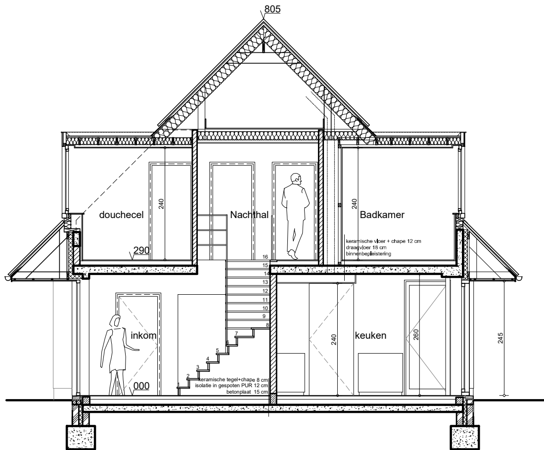
Doorsnede C
