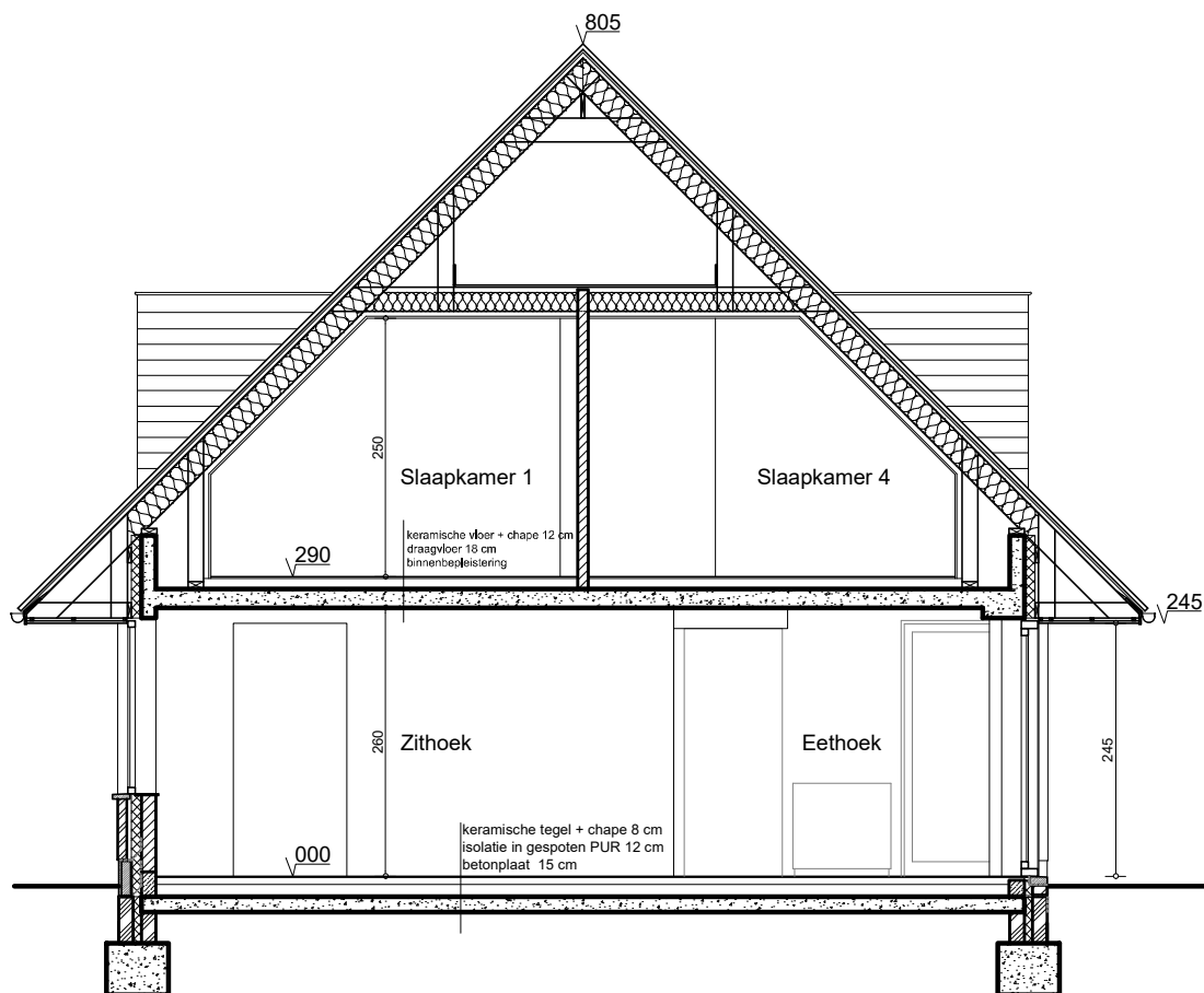
Doorsnede E
