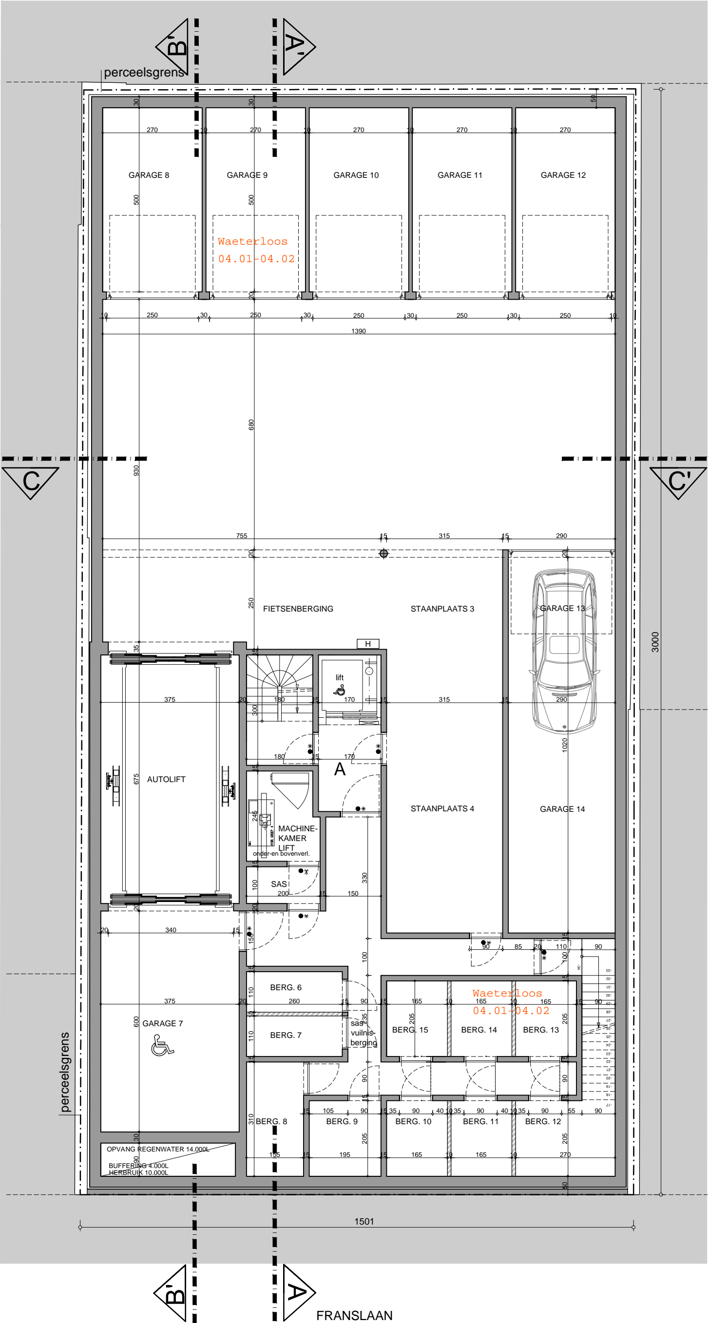
NIVEAU -2 schaal 1|100
