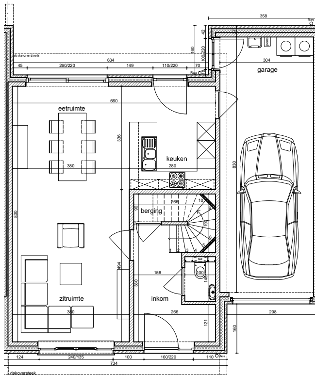
LOT 28 - GELIJKVLOERS
